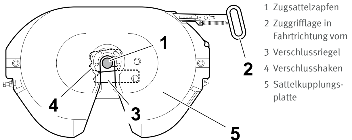
Abb. 8 Bauteile und Funktionsprinzip der Sattelkupplung
