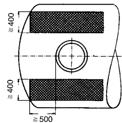
Doppelter Laufsteg
