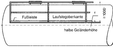
Laufsteg mit feststehendem Geländer
